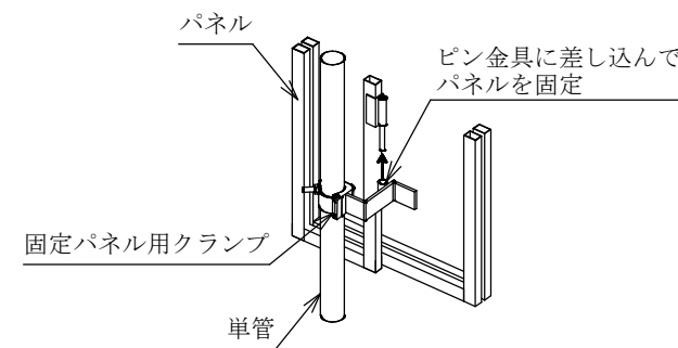
C部詳細図
