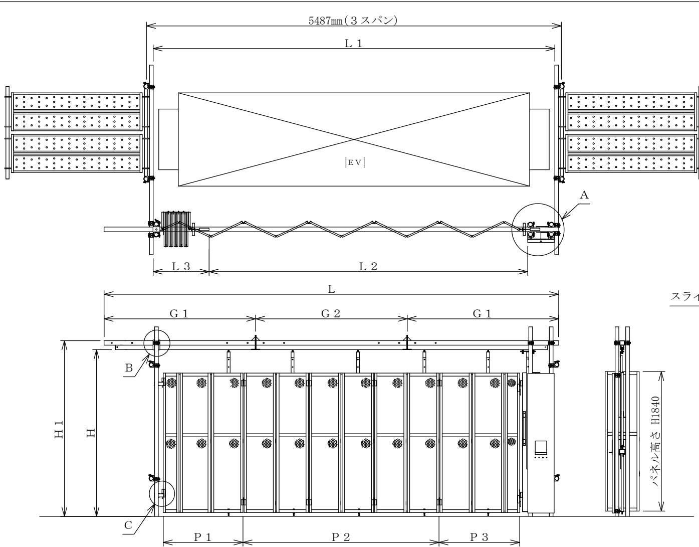
SPP-5.4型正面図 (図は3スパン用)
